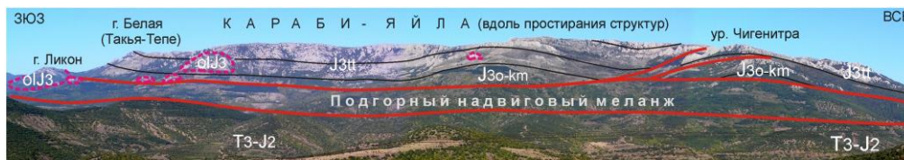
Рис. 8. Строение южного края Карабийского массива.
