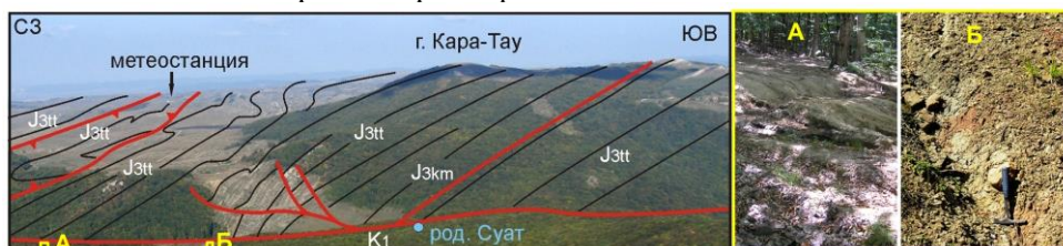
Рис. 5. Стрoение правого берега истоков р. Суат из известняков и песчаников верхней юры, подстилаемых через пологий надвиг толщeй нижнего мела. Фото А – размокающие глины в колее дороги, Б – меланжированные глины в промоине у дороги на склоне.
