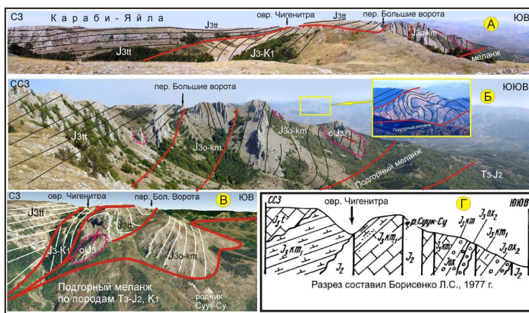
Рис. 10. Фронтальные структуры юго-восточной части Карабийского массива.
